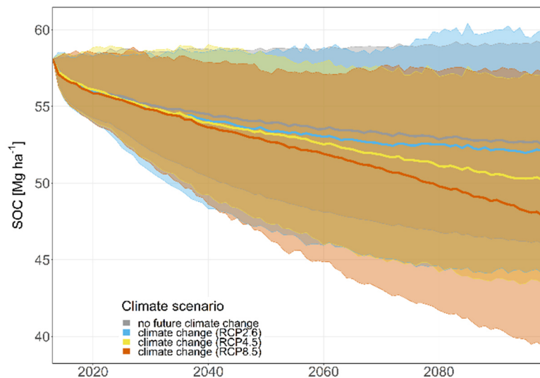
Abbildung 1: Entwicklung mittlerer Bodenkohlenstoffvorräte auf Ackerland in Deutschland unter Beibehaltung aktueller C-Einträge, dargestellt als Mittel der Ensemble-Modellierungen von mindestens fünf regionalen Klimamodellen und fünf Bodenkohlenstoff-Modellen mit 95-Prozent-Konfidenzintervall unter der Annahme von vier verschiedenen Klimaszenarien [37].
